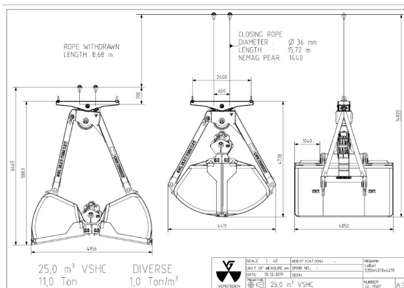
Εικόνα 4: Σχεδίου Αρπάγης Χύδην Φορτίου Μικτού Βάρους 36t.
