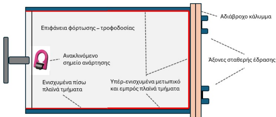
Εικόνα 3: Κάτοψη ρυμουλκούμενης διάταξης σε Κατάσταση Μεταφοράς.
